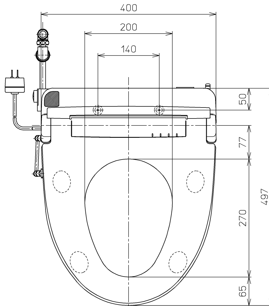
便器洗浄コード L=1200
